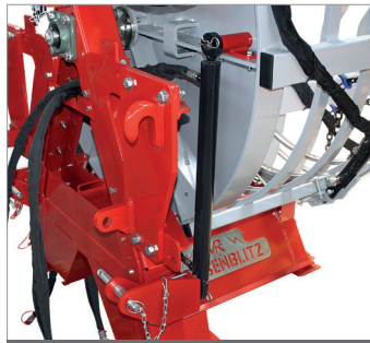
Hydraulisch kippbar
